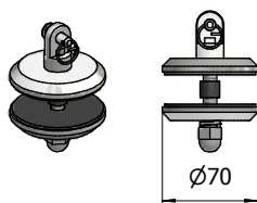
Supporto vetro per il tirante
