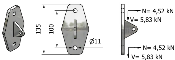
Supporto vetro per il tirante
