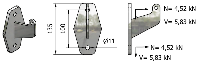
Supporto vetro per fissaggio inferiore
